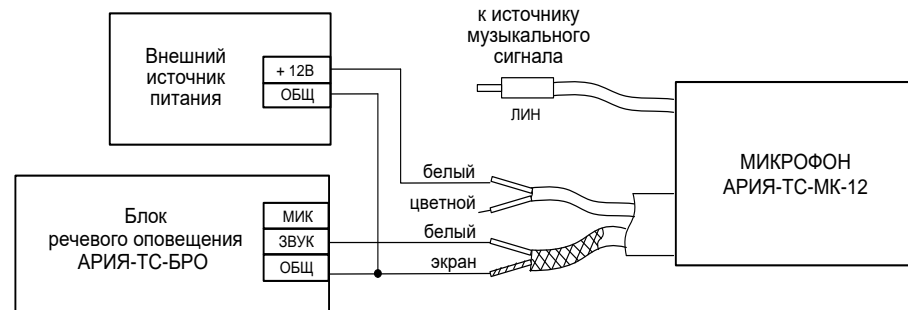
Рис.2. Схема соединений при подключении микрофона с минимальным приоритетом.
