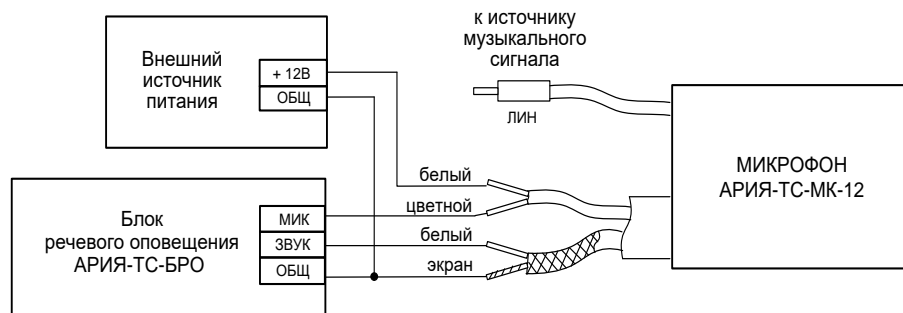
Рис.1. Схема соединений при подключении микрофона с максимальным приоритетом.
